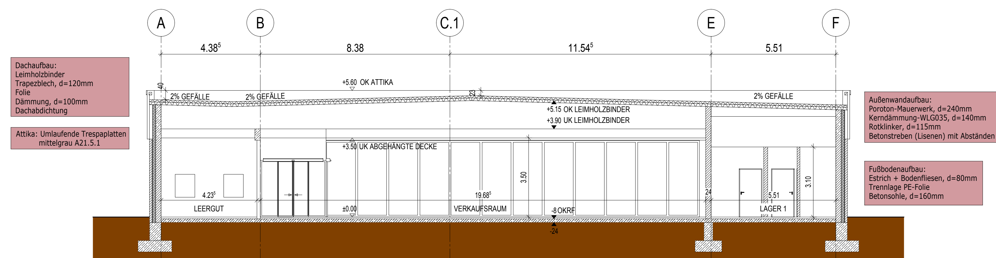
- SCHNITT B-B -
