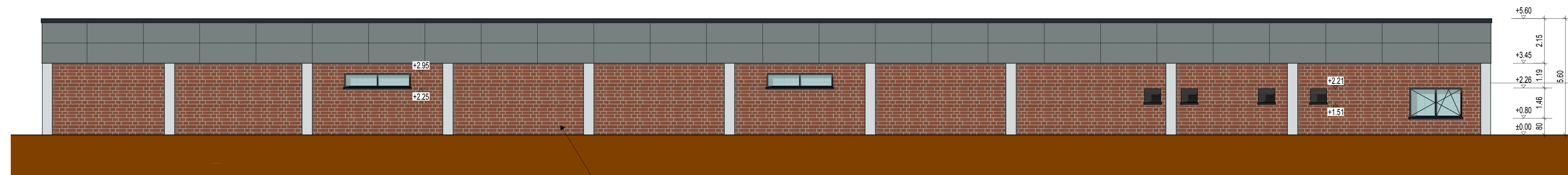
- Ansicht Westen -
